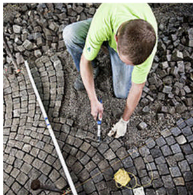
Paveur CFC
